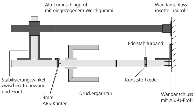
Zeichnung: Kabinenanlage Typ SVF30 JUMP
