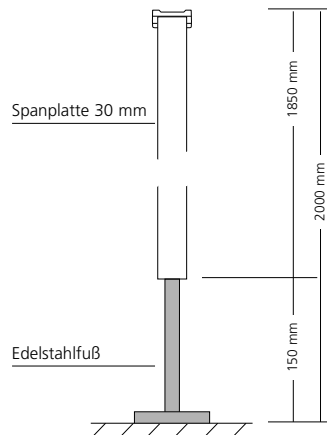
Zeichnung: Schnitt
