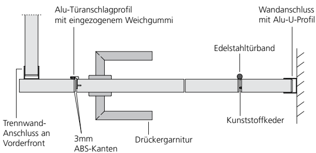
Zeichnung: Kabinenanlage Typ SVF30
