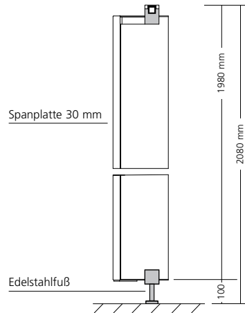
Zeichnung: Schnitt
