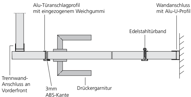
Zeichnung: Kabinenanlage Typ SV30
